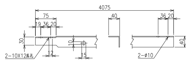
胴縁 S=1/4
