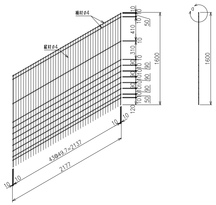
動物侵入防止柵用クリップ金網 S=1/20
