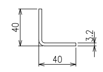
胴縁 S=1/2
