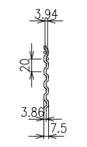
0部詳細図 S=1/4
