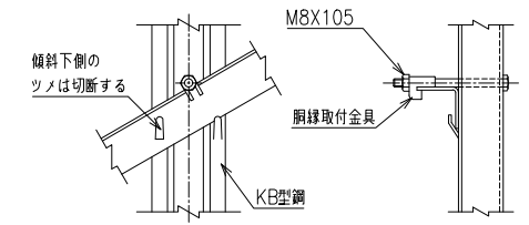
主柱胴縁取付詳細図 S=1/4
