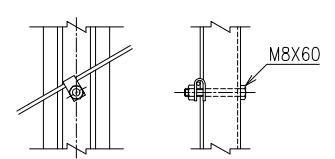
主柱骨線取付部 S=1/4
