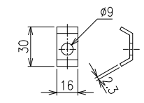
胴縁用金網取付金具 S=1/2
