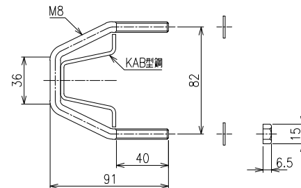
Uボルト、ナット S=1/2
