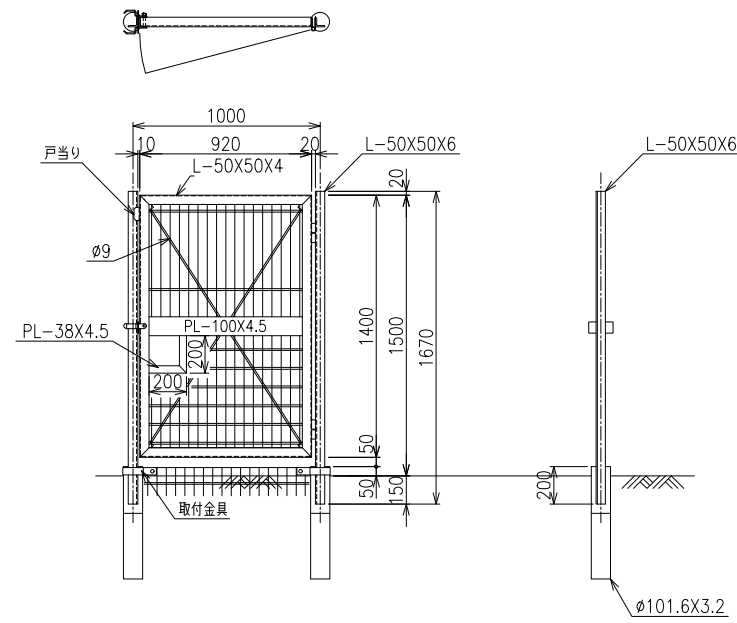
片開き門扉 S=1/20
