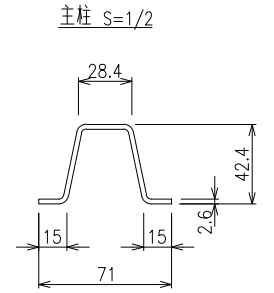
胴縁 S=1/2
