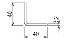
端柱 S=1/2
