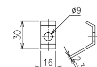
胴縁用金網取付金具 S=1/2
