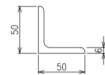
端柱 S=1/2
