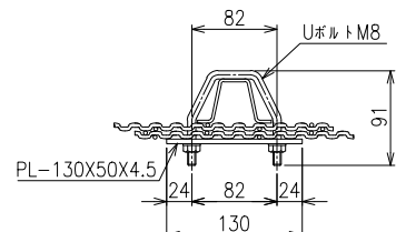
A部詳細図 S=1/4
