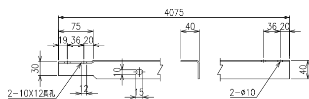
胴縁 S=1/4
