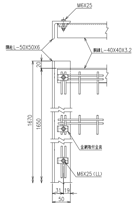
胴縁 S=1/4
