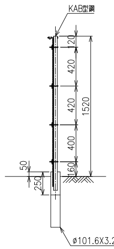
側面図 S=1/20
