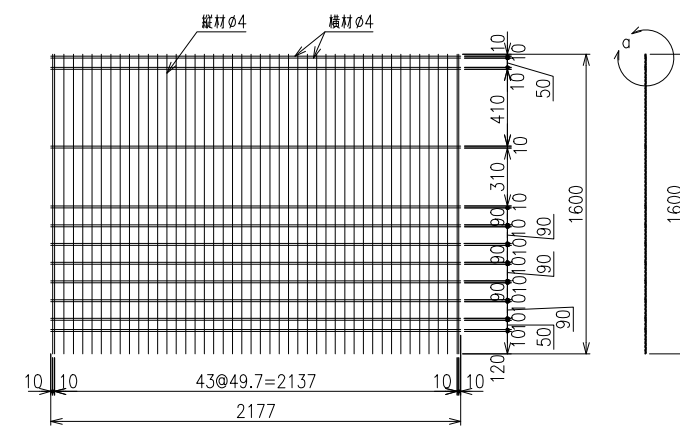
動物侵入防止柵用クリップ金網 S=1/20
