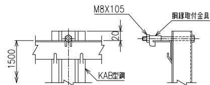
主柱胴縁取付詳細図 S=1/4
