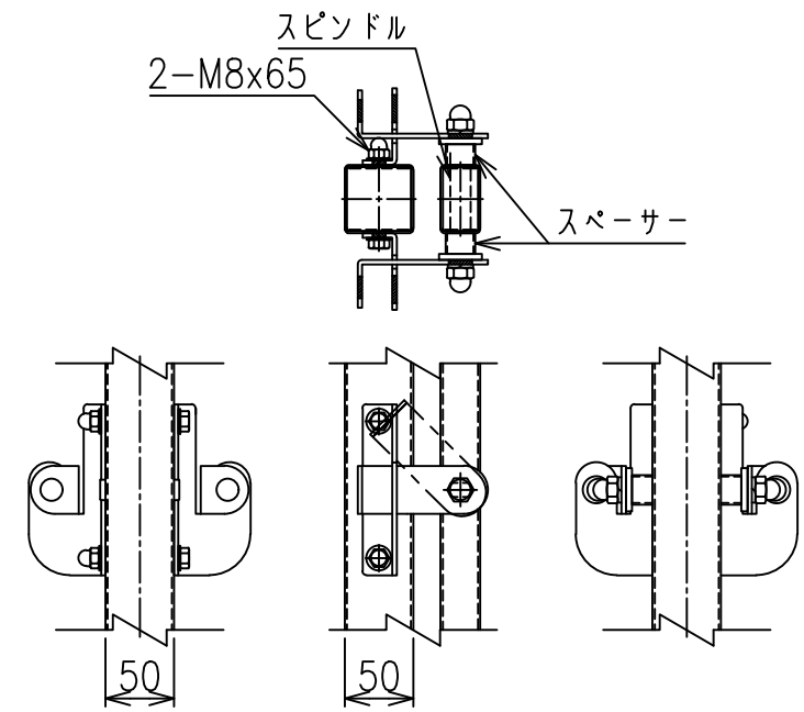
B部詳細図 S=1/6
