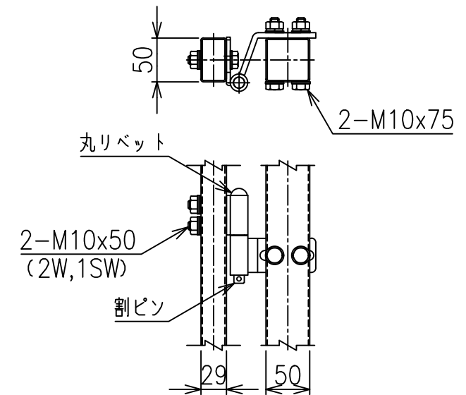
B部詳細図 S=1/6
