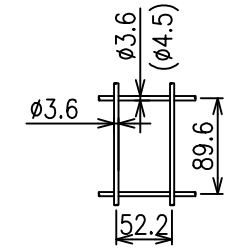
メッシュ寸法図 S=1/5
