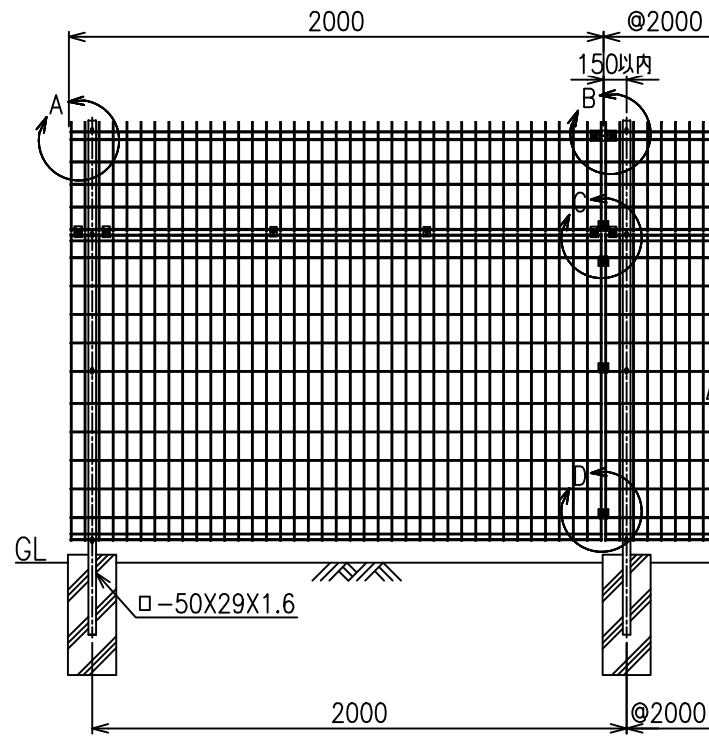
正面図 S=1/20
