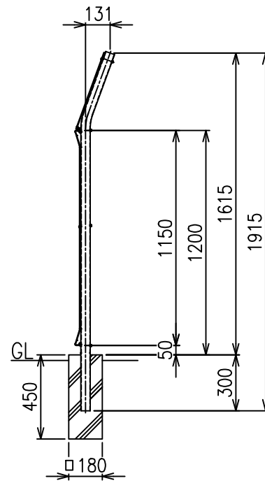
側面図 S=1/20
